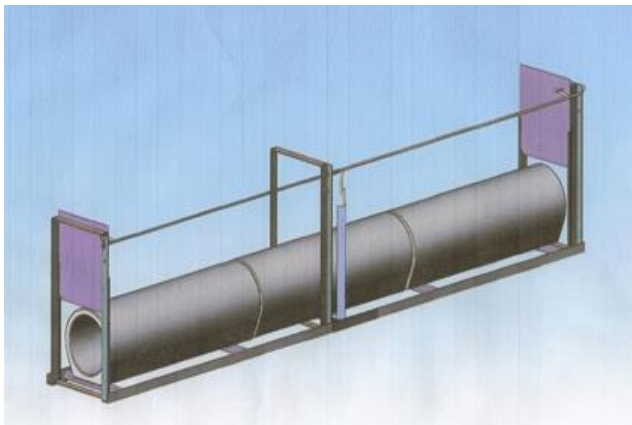
Betonrohrfalle
